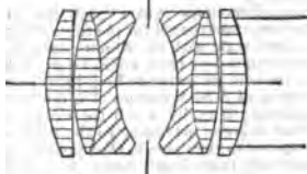
FIG. 43.—Planar. Series Ia. f/4 .
