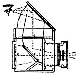
FIG. 10.—Reflex Camera.
