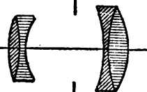
FIG. 58.—"Bis-Telar."
