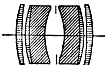
FIG. 54.—Euryplan, f/4.5 .
