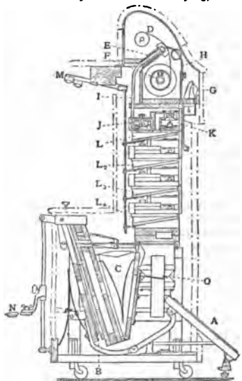
FIG. 36.—Modern Pianola.
